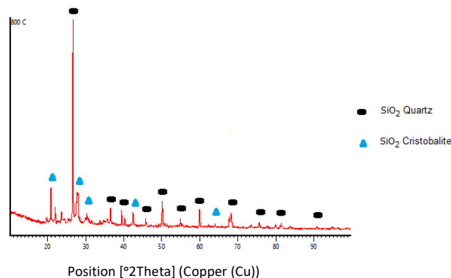
Gambar 4 Hasil XRD Silika dengan Temperatur Kalsinasi 800 °C
