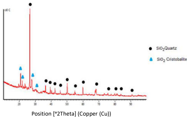
Gambar 3 Hasil XRD Silika dengan Temperatur Kalsinasi 700 °C
