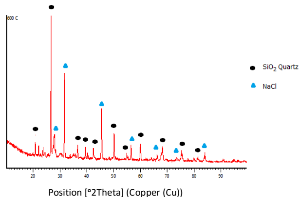
Gambar 2 Hasil XRD Silika dengan Temperatur Kalsinasi 600 °C
