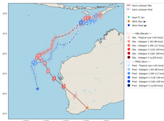
Gambar 4 Visualisasi prediksi (biru) trajektori dan intensitas terhadap observasi (merah) pada Siklon Tropis Seroja
