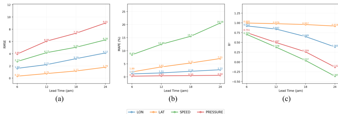
Gambar 3 Evaluasi prediksi intensitas dan lintasan Siklon Tropis Seroja menggunakan (a) RMSE, (b) MAPE, dan (c) R^2
