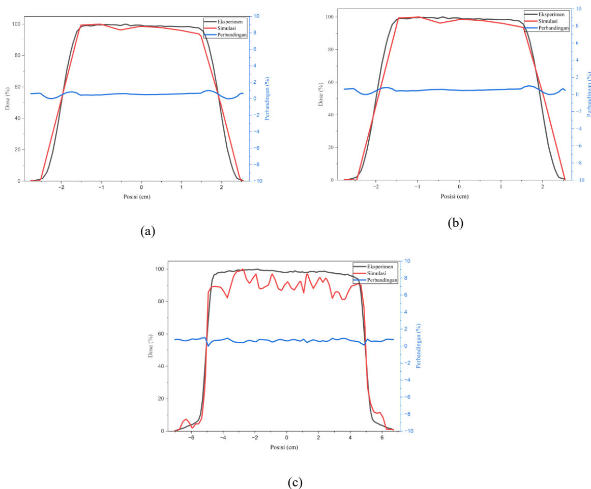
Gambar 2 Perbandingan hasil eksperimen dengan simulasi dose profile (a) kedalaman 1,5 cm (b) kedalaman 5 cm (c) kedalaman 10 cm
