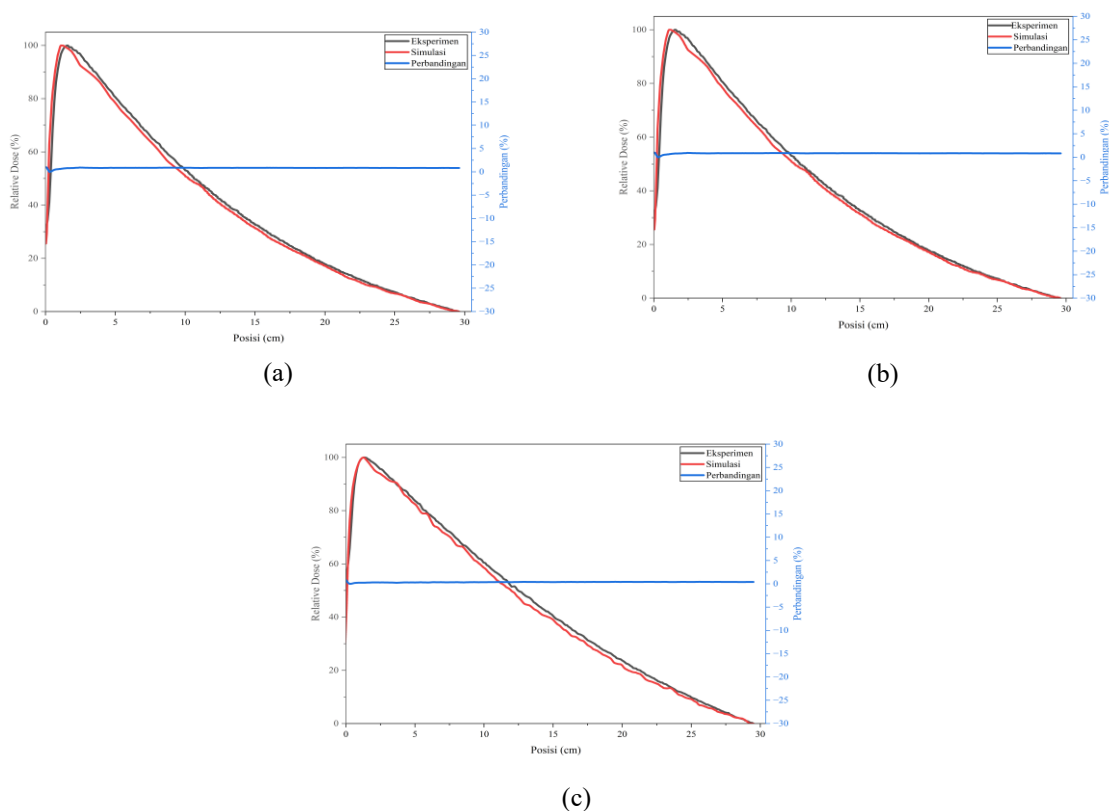
Gambar 1 Perbandingan hasil eksperimen dan simulasi PDD ukuran lapangan (a) ( 4 \times 4 ) \text{cm}^2 , (b) ( 10 \times 10 ) \text{cm}^2 , dan (c) ( 40 \times 40 ) \text{cm}^2
