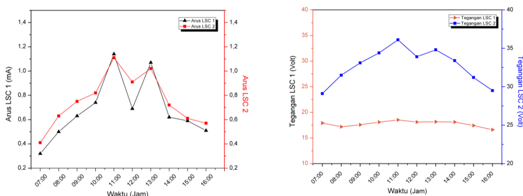
Gambar 6 (a) Grafik Arus (mA) (b) Grafik Tegangan (Volt)
