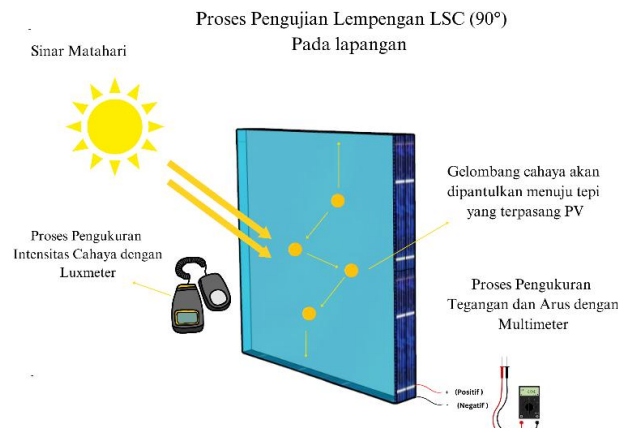
Gambar 3 Proses pengujian sampel LSC-PV di lapangan
