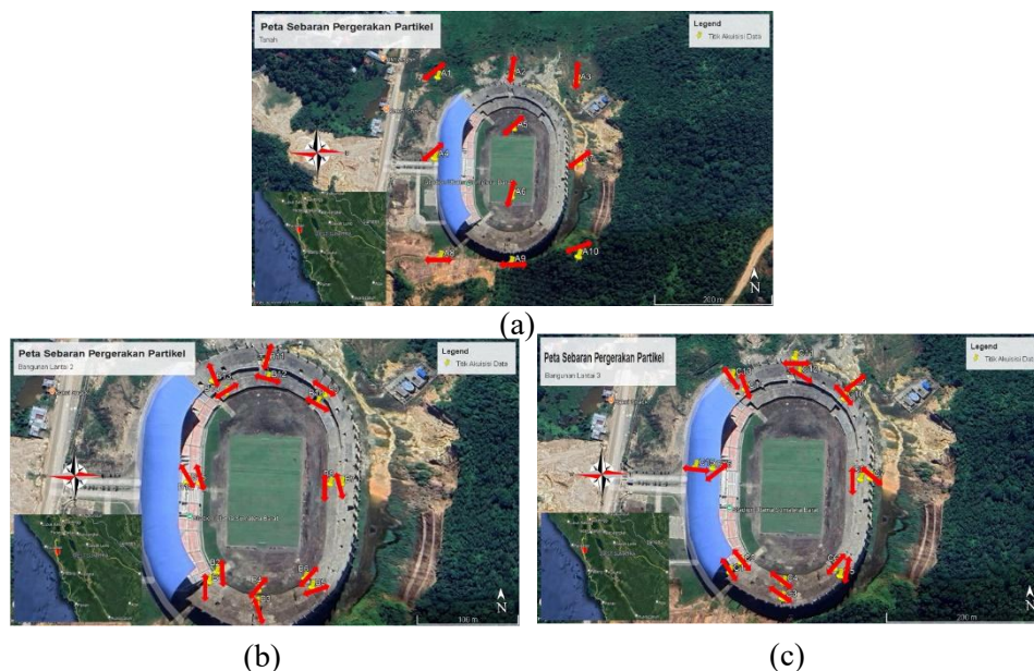
Gambar 5 Peta sebaran arah pergerakan partikel: (a) tanah, (b) bangunan lantai 2 dan (c) bangunan lantai 3
