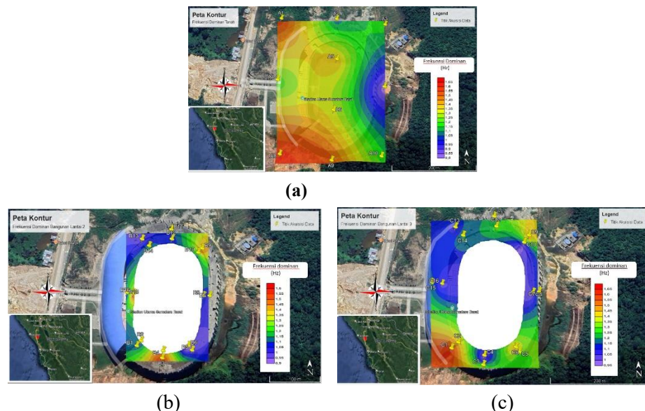
Gambar 2 Peta sebaran frekuensi dominan: (a) pada tanah, (b) pada bangunan lantai 2 dan (c) pada bangunan lantai 3
