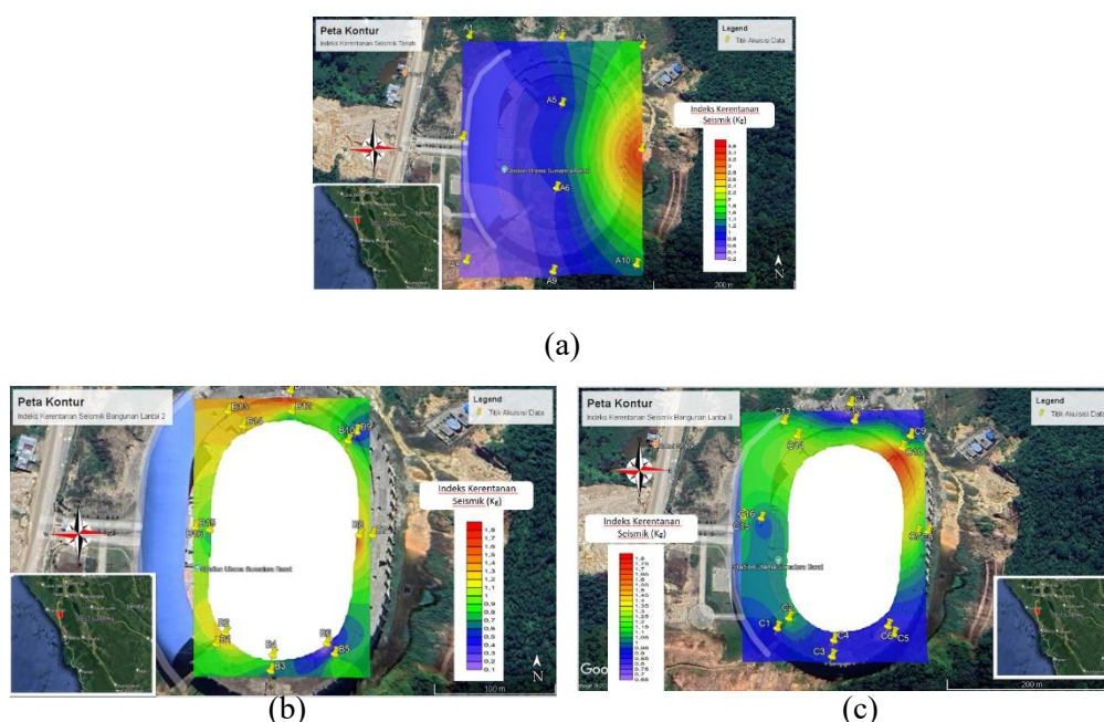
Gambar 4 Peta sebaran indeks kerentanan seismik: (a) pada tanah, (b) pada bangunan lantai 2 dan (c) pada bangunan lantai 3
