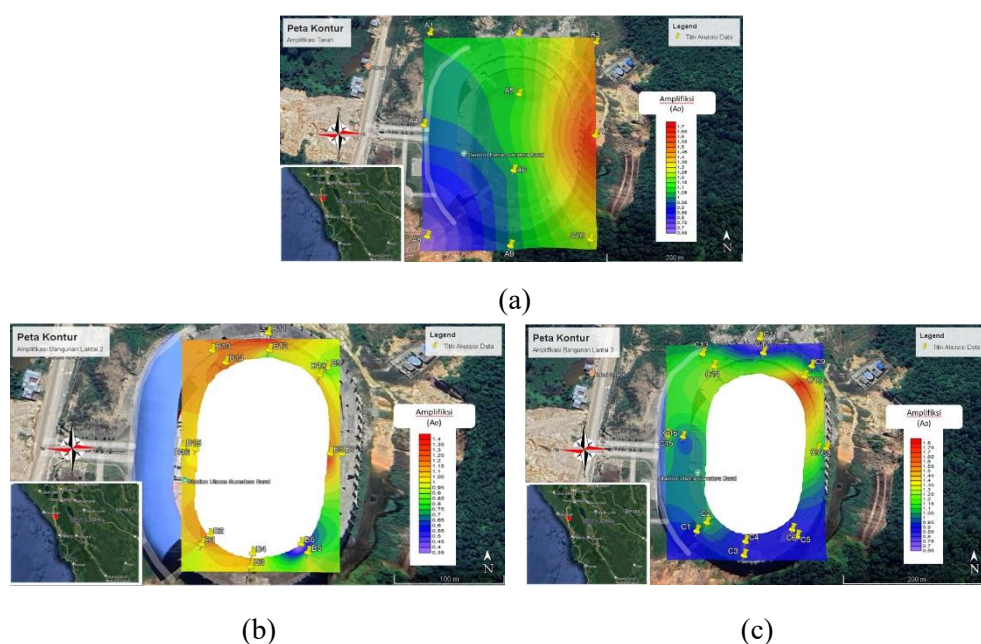
Gambar 3 Peta sebaran amplifikasi: (a) tanah, (b) bangunan lantai 2 dan (c) bangunan lantai 3
