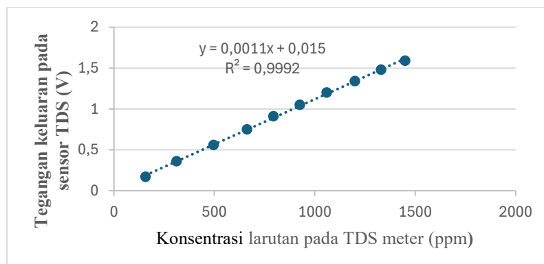
Gambar 4 Hubungan antara konsentrasi larutan dengan Tegangan Keluaran Sensor
