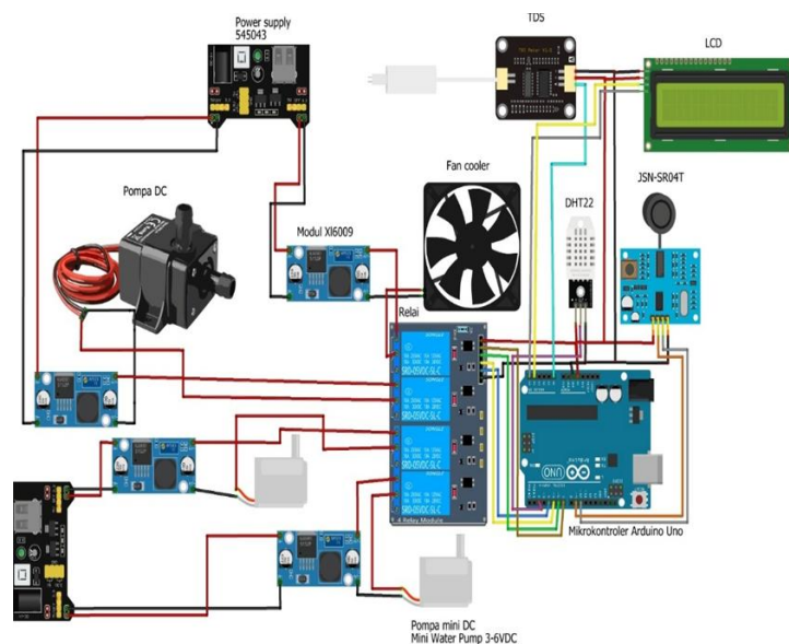
Gambar 2 Rangkaian Sistem Secara Keseluruhan
