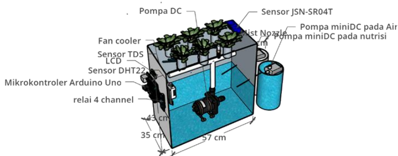
Gambar 6 Alat Keseluruhan
