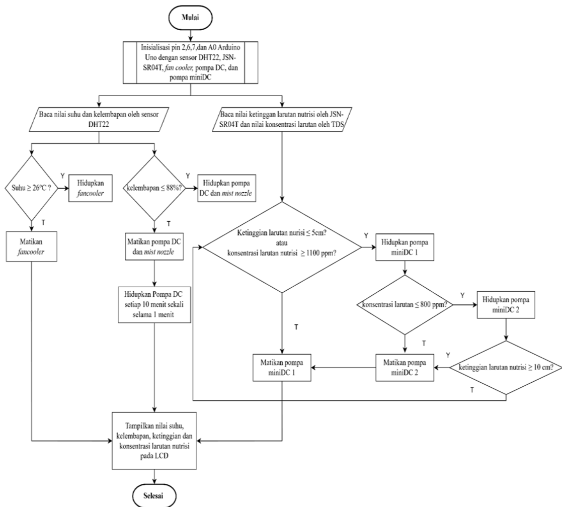
Gambar 3 Diagram Alir Perangkat Lunak Sistem
