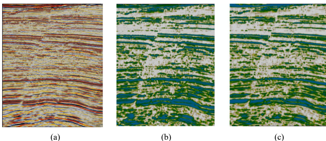
Gambar 3 Hasil pelatihan JST kombinasi atribut pada crossline 1271 (a) Penampang Awal (b) Kombinasi 5 atribut (c) Kombinasi 3 atribut
