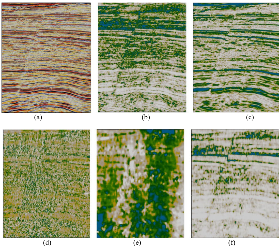
Gambar 2 Hasil pelatihan JST satu atribut pada Crossline 1271 (a) penampang awal (b) similarity (c) spectral decomposition (d) curvature (e) dip (f) semblance
