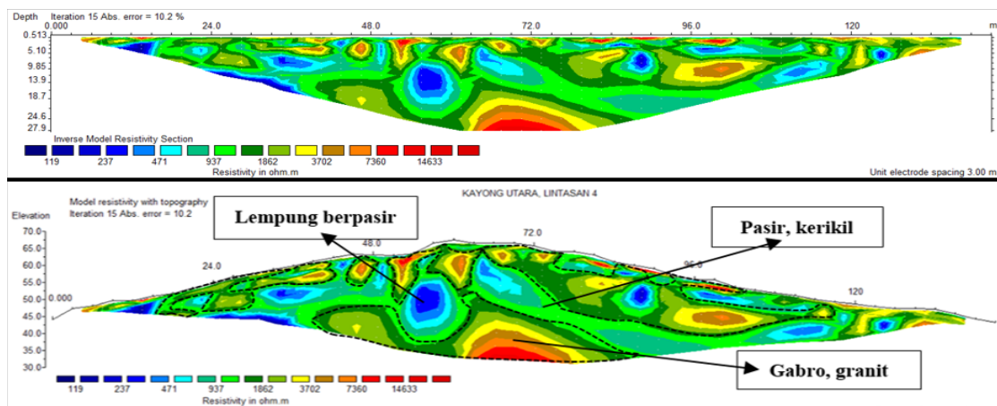
Gambar 7 Penampang hasil resistivitas 2D lintasan keempat
