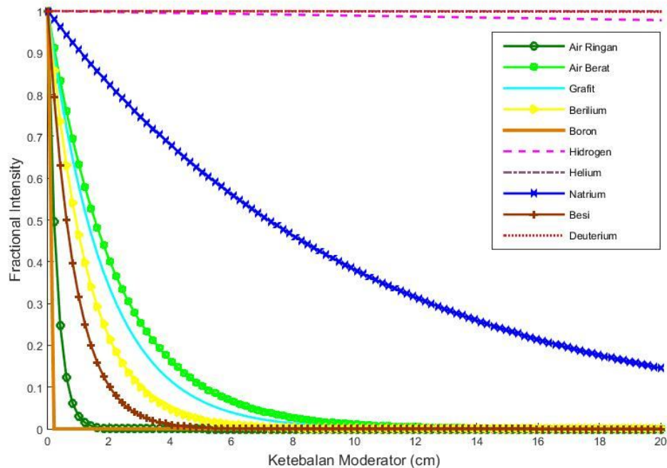
Gambar 1 Grafik faktor pelemahan neutron pada 10 bahan
