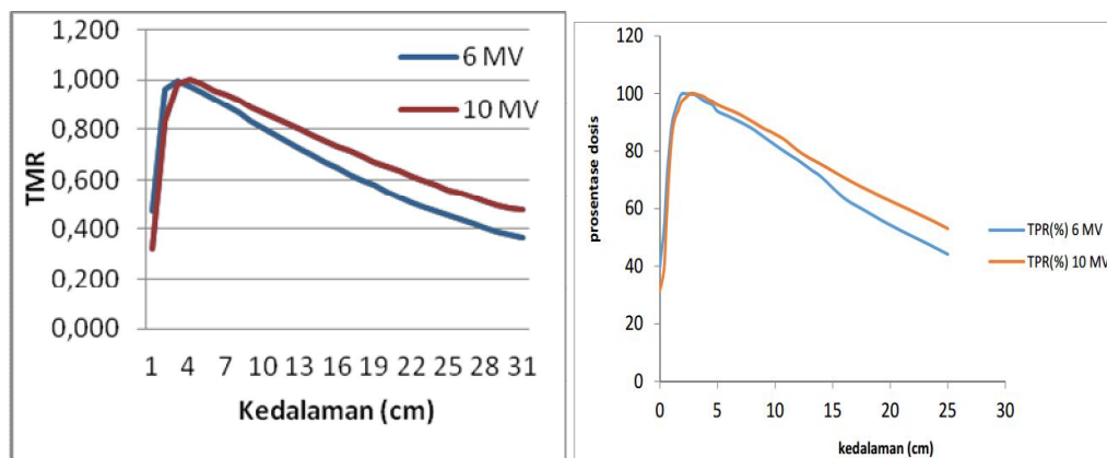
Gambar 4 (a) Hasil pengukuran TMR energi 6 MV dan 10 MV untuk lapangan (9x9) cm 2 dari hasil penelitian (b) Nilai TPR energi 6 MV dan 10 MV (sumber: Laksono dkk, 2015)
