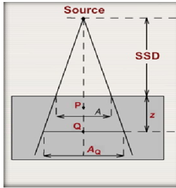
Gambar 1 Teknik penyinaran SSD
