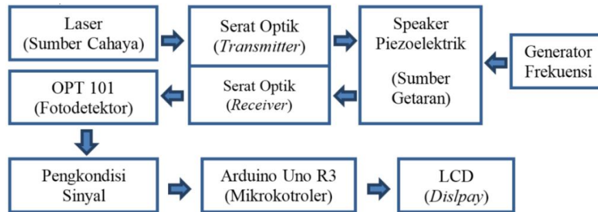
Gambar 2. Skema Perangkat Keras Sistem Pengukuran Frekuensi Getaran Akustik Menggunakan Sensor Serat Optik
