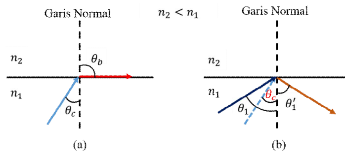
Gambar 1 (a) Sudut datang sebesar \theta_c (b) Sudut datang lebih besar dari \theta_c
