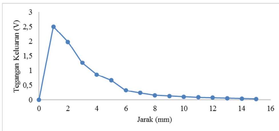
Gambar 4. Grafik Perubahan Jarak antara Elemen Speaker dan Serat Optik terhadap Tegangan Keluaran Fotodiode OPT101
