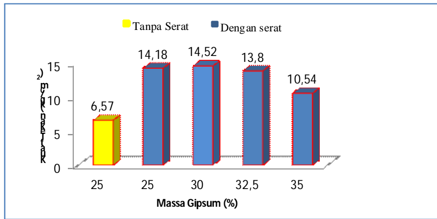
Gambar 1 Pengaruh massa gipsium terhadap kuat tekan dengan serat tetap 2,5%
