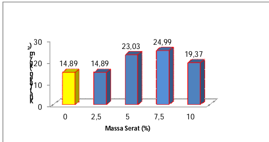
Gambar 2 Pengaruh massa serat terhadap kuat tekan dengan gipsium tetap 30%
