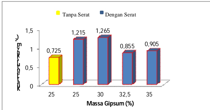
Gambar 3 Pengaruh massa gipsium terhadap kuat lentur dengan serat tetap 2,5%
