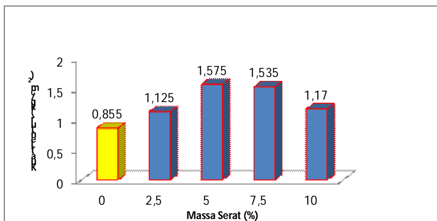
Gambar 4 Pengaruh massa serat terhadap kuat lentur dengan gipsium tetap 30%
