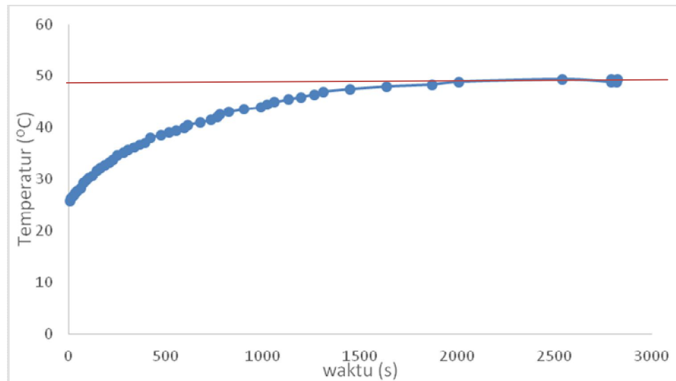
Gambar 6 Grafik hubungan temperatur terhadap waktu pada sistem kontrol temperatur air pada proses pemanasan
