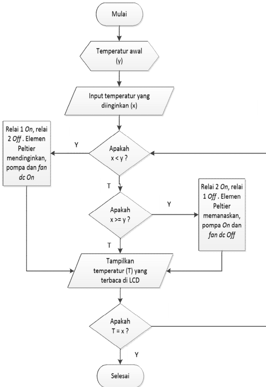
Gambar 2 Diagram alir perangkat lunak sistem kontrol temperatur
